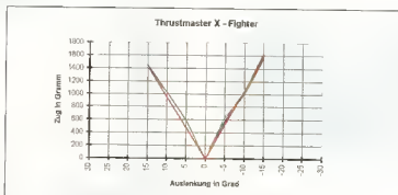
Optimaler Verlauf für einen Joystick mit mehr als 2 kg Zug.
